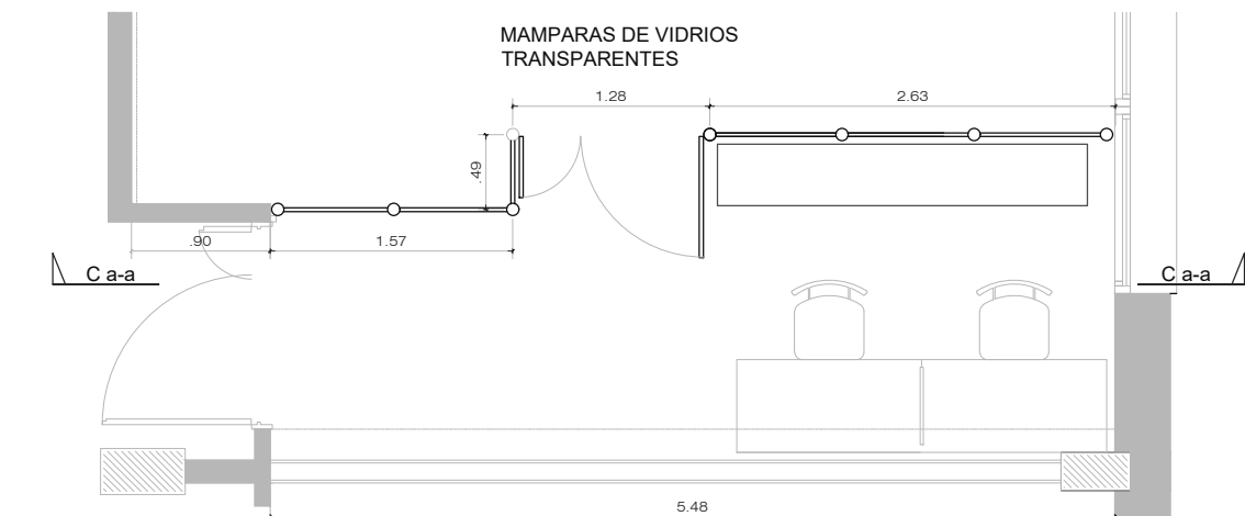
planta; Esc. 1:50
