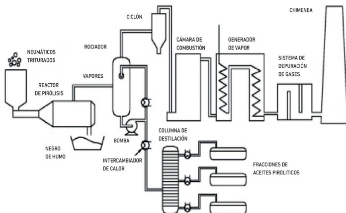
Figura A1F3 Proceso de pirólisis
