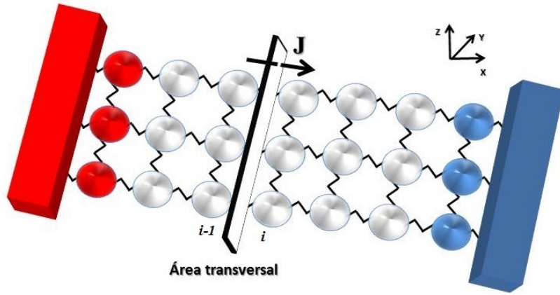
Figura 11: Esquema de la lámina y de una sección transversal por donde fluiría la corriente térmica de izquierda a derecha de la misma. La corriente será la suma de las corrientes de todo enlace individual que atraviese dicha superficie.
