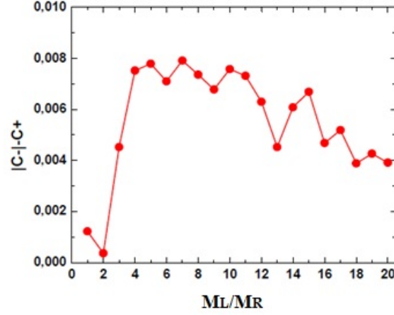
Figura 17: Diferencias en las conductancias como una función del cociente de las masas M_L/M_R . (N_x, N_y) = (20, 20) , T_L = 1.5 \cdot 10^{-6} , T_R = 5 \cdot 10^{-7} , a_x = 1.10 .
