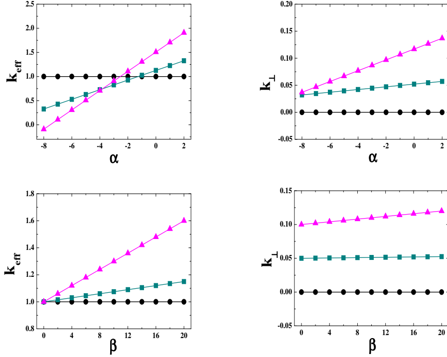
Figura 21: Constante elásticas efectivas: Longitudinal ( k_{\text{eff}} ) y Transversal ( k_{\perp} ), como función de \alpha para \beta = 16.93 (fila superior) y como función de \beta para \alpha = 0 (fila inferior). En todos los casos k_2 = 1.0 y l_o = 1.0 . \epsilon = 0 (puntos negros), \epsilon = 0.05 (cuadrados cian oscuro) y \epsilon = 0.1 (triángulos magenta).
