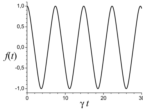
Figura 30: Solución temporal de f(t) .
