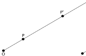
Homotecia de centro O y razón 3
