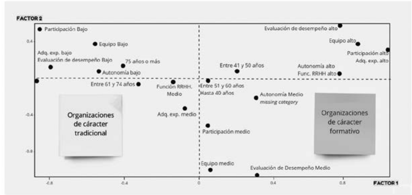
Figura 2. Representación de ejes factoriales, variables activas y variables suplementarias seleccionadas
