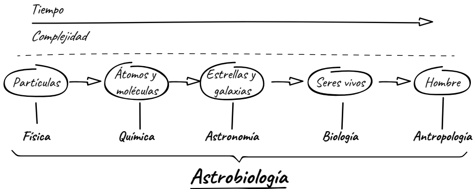
Figura 1. La astrobiología como una disciplina integradora
