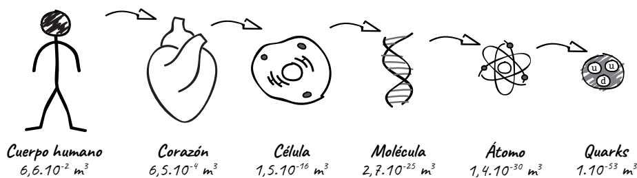
Figura 3. Relación de tamaño entre los distintos componentes de la realidad física
