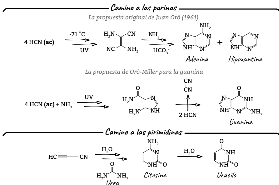
Figura 28. Posibles caminos químicos de obtención de las purinas y pirimidinas
