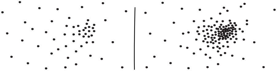
Figura 12. Representación del proceso de aumento de la densidad del gas interestelar por acción de la fuerza de gravedad
