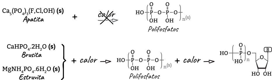
Figura 34. Formación de nucleótidos a partir de nucleósidos
