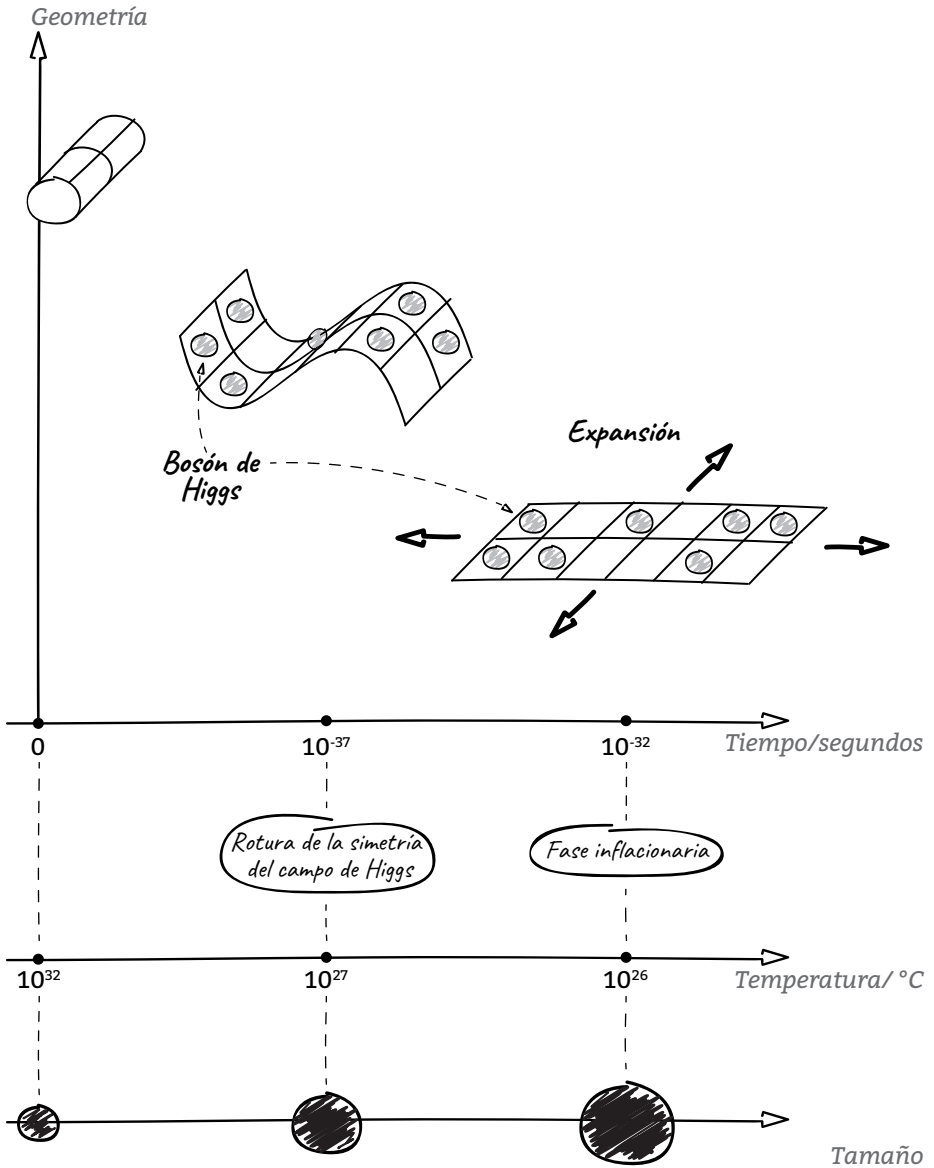
Figura 4. Etapa inflacionaria en una representación bidimensional (el eje del tamaño solo indica al aumento de este)
