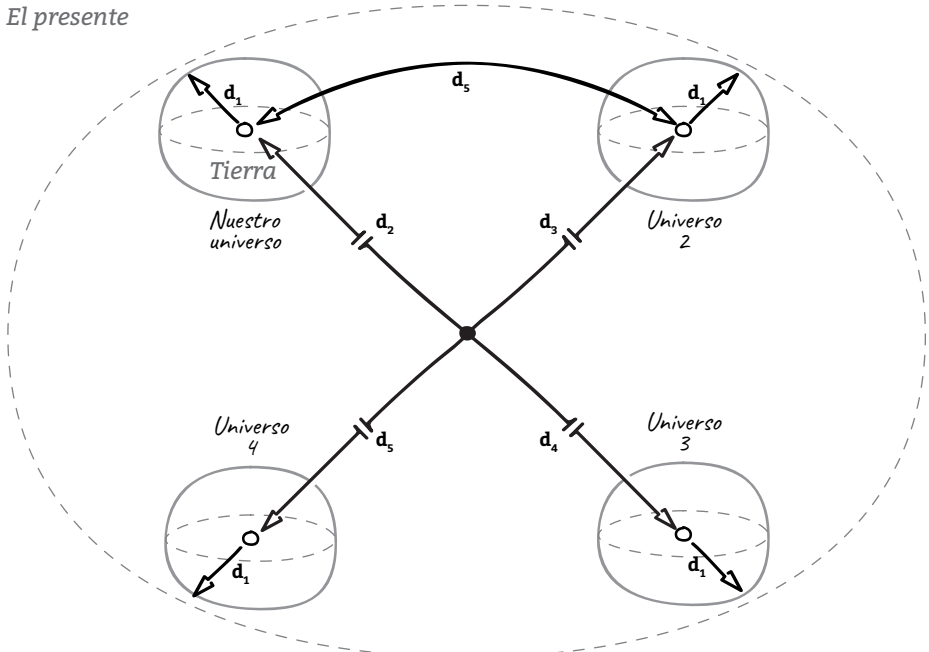
Figura 77. Representación de múltiples universos desconectados
