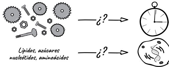
Figura 35. La analogía reloj-célula
