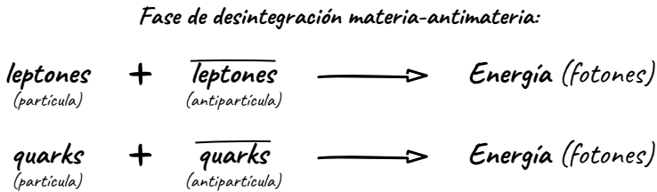
Figura 7. Transformaciones de la etapa de desintegración materia-antimateria
