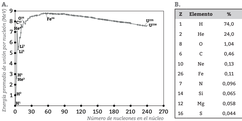
Figura 13b. Representación del proceso de nucleosíntesis en una estrella.
