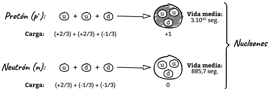
Figura 8. Formación de los nucleones a partir de los quarks
