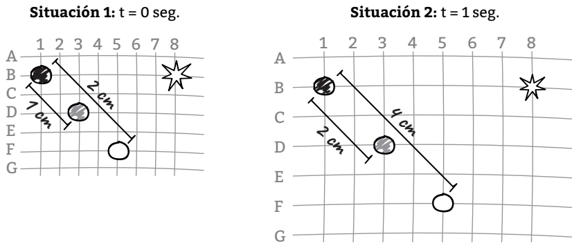
Figura 2. Expansión de un plano sin centro de expansión (Big Bang en el plano)
