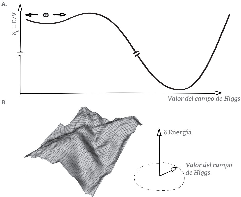
Figura 76. La idea de múltiples valores escalares de Higgs en diversos universos
