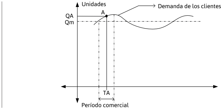
Figura 5.1. Gráfico de la demanda continua
