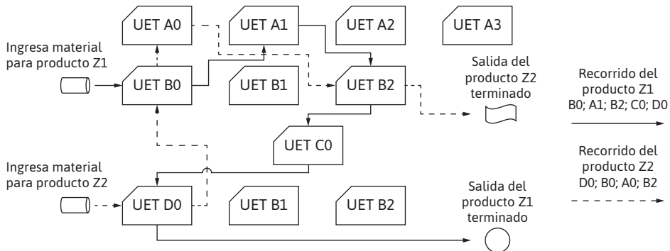
Figura 4.2. Disposición de las UET por principio de realización o proceso, vinculación lógica
