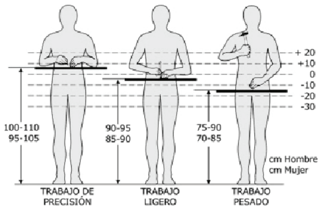
Figura 17.11. Dimensiones de los puestos para la posición de pie haciendo referencia al tipo de tarea
