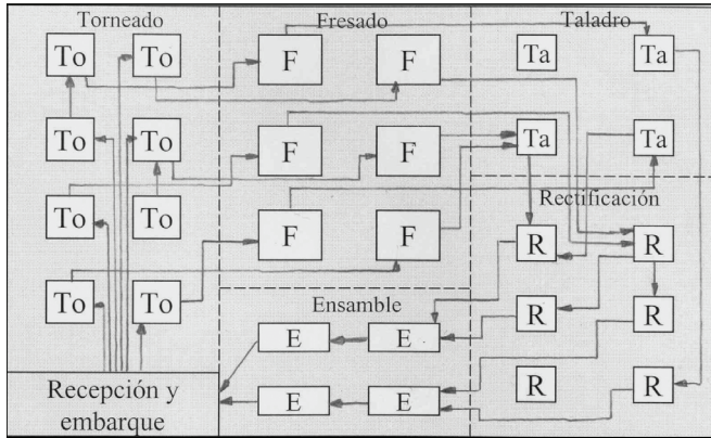
Figura 16.5. Taller en típica distribución por proceso
