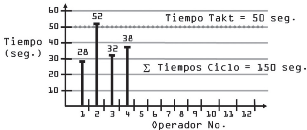
Figura 16.13. Gráfico de tiempos de una célula de fabricación con cuatro operarios
