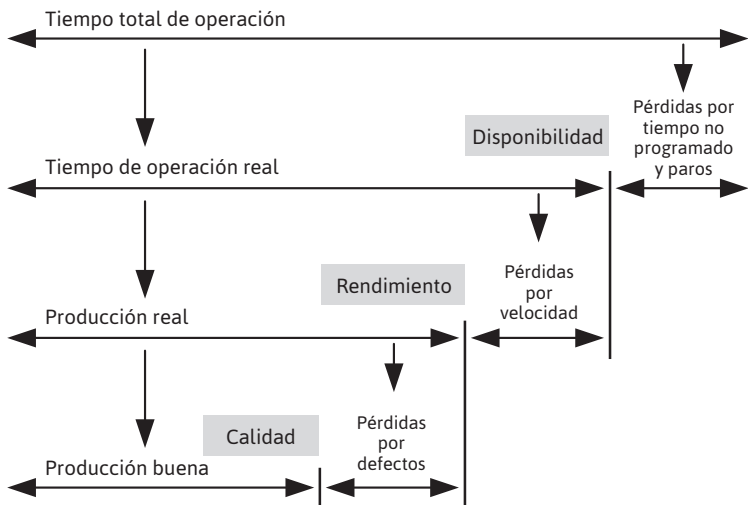
Figura 8.6. Medición de efectividad de equipos
