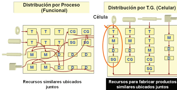
Figura 16.8. De una distribución por proceso a una distribución por tecnología de grupo (celular)
