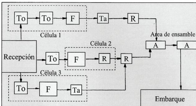
Figura 16.6. Taller en típica distribución de tecnología de grupo
