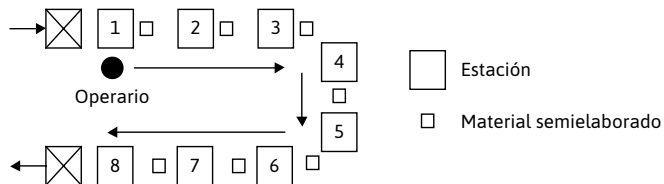
Figura 16.12. Célula de armado con un operario
