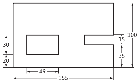
Figura 13.2. Pieza a la cual se le conocen los tiempos, tabulados en la tabla 13.1
