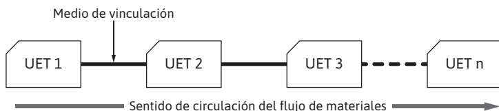
Figura 4.1. Disposición de las UET por principio de flujo, vinculación física
