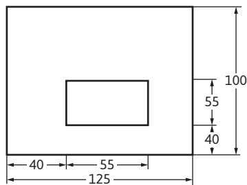
Figura 13.1. Pieza para el cálculo del tiempo por comparación en el ejemplo didáctico
