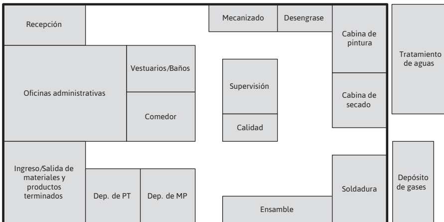
Figura 16.16. Diagrama de bloques de una planta industrial (sin detalle de máquinas)
