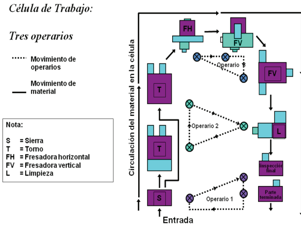
Figura 16.10. Célula de trabajo con tres operarios
