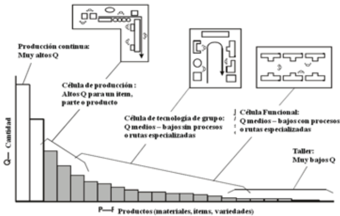
Figura 16.11. Tipos de células de trabajo según P (variedad de productos), Q (cantidad) y R (rutas de fabricación/armado)
