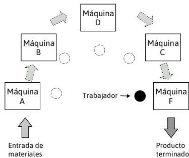
Figura 16.7. Esquema de una célula OWMM
