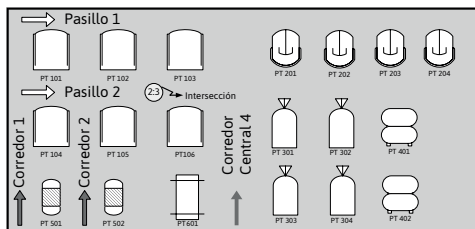
Figura 10.3. Sobre un layout de la planta se indican los pasillos y corredores de circulación, así como la disposición de los puestos de trabajo
